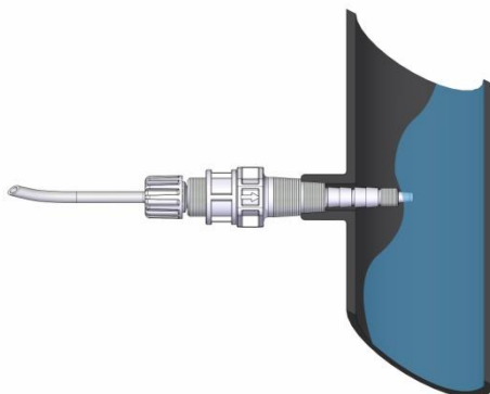
INSTALLATION SU ATTACCO 3/8"
